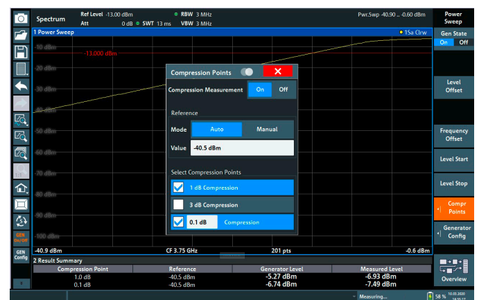
Измерение точек компрессии 1 дБ и 0,1 дБ
