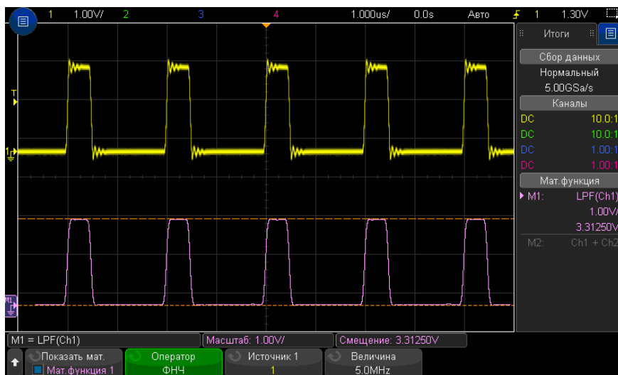
Рис. 16 Пример фильтра низких частот
