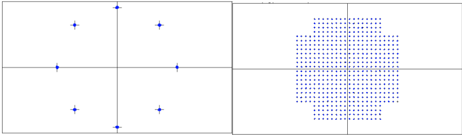
Fig. 2.9 8PSK
