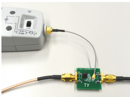
Рисунок 6а. Кабель SMA
