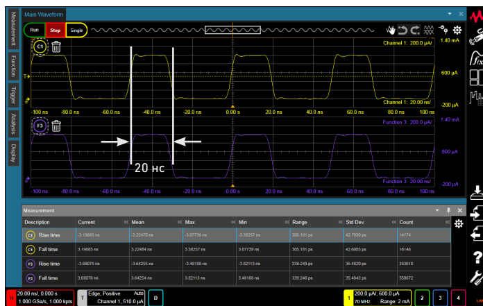
Рисунок 9. Возможность с легкостью измерять переходные токи с шириной импульса менее 100 нс, что поможет при оценке и анализе таких двухполюсных элементов, как PRAM, ReRAM, MRAM и др.
