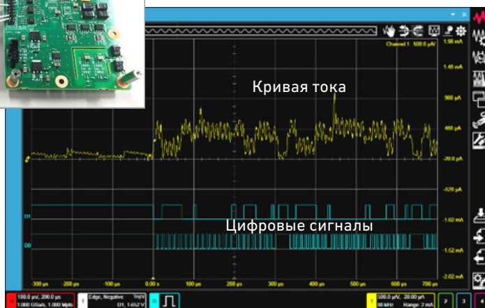
Рисунки 14a, 14b. Пример измерения кривой тока и соединения с помощью цифрового канала.
