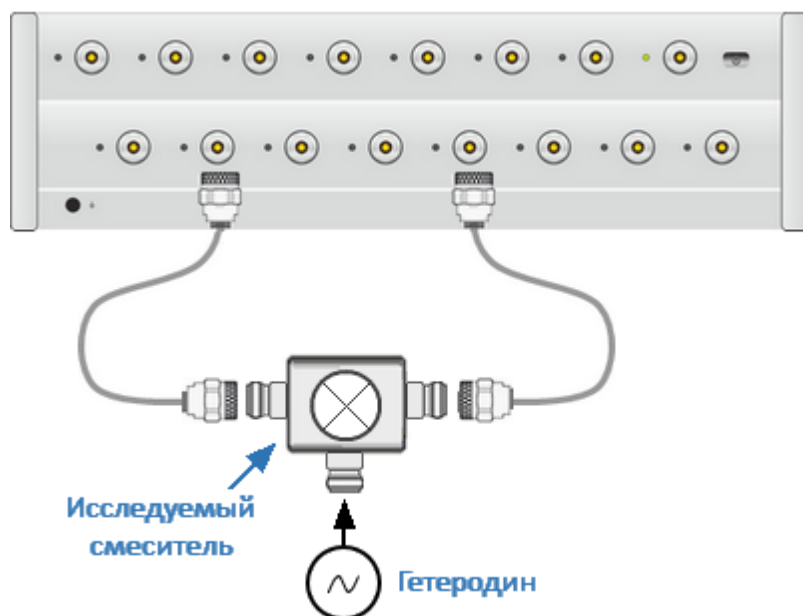
Рисунок 173 — Схема скалярного измерения смесителя
