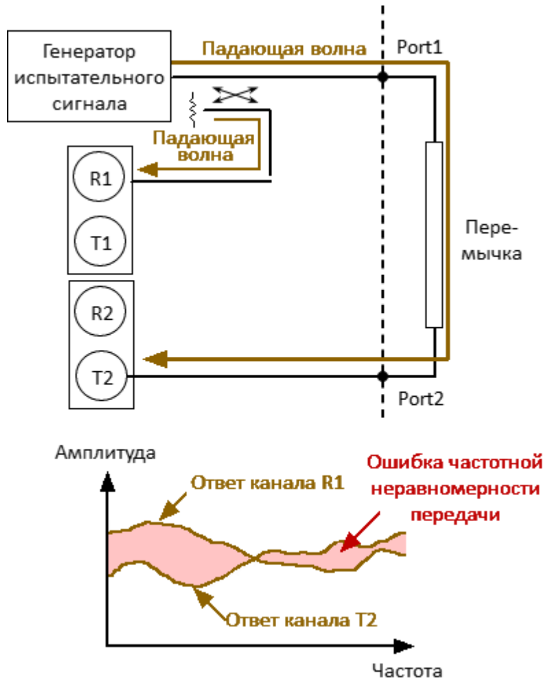
Рисунок 78 — Ошибка частотной неравномерности передачи
