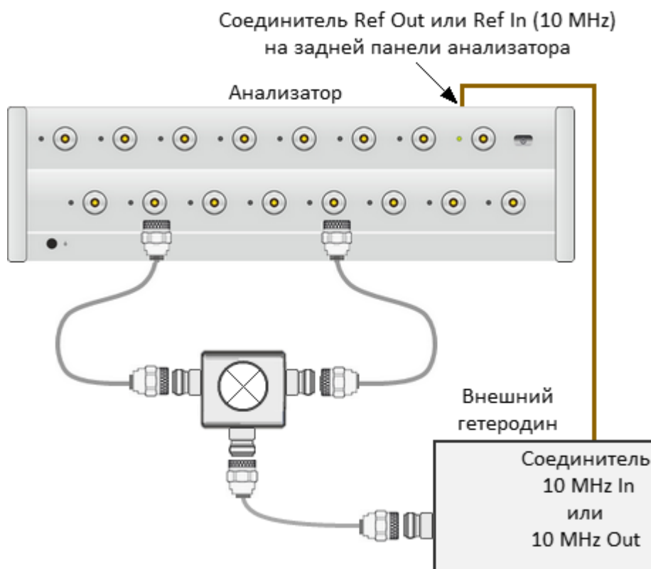
Рисунок 179 — Синхронизация анализатора и внешнего гетеродина по опорной частоте
