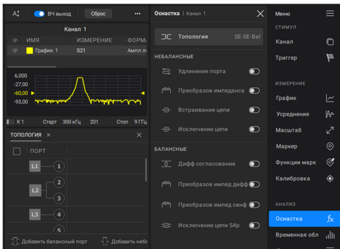
Рисунок 150 — Пример топологии
