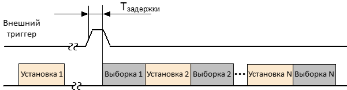
Рисунок 58 — Задержка внешнего триггера
