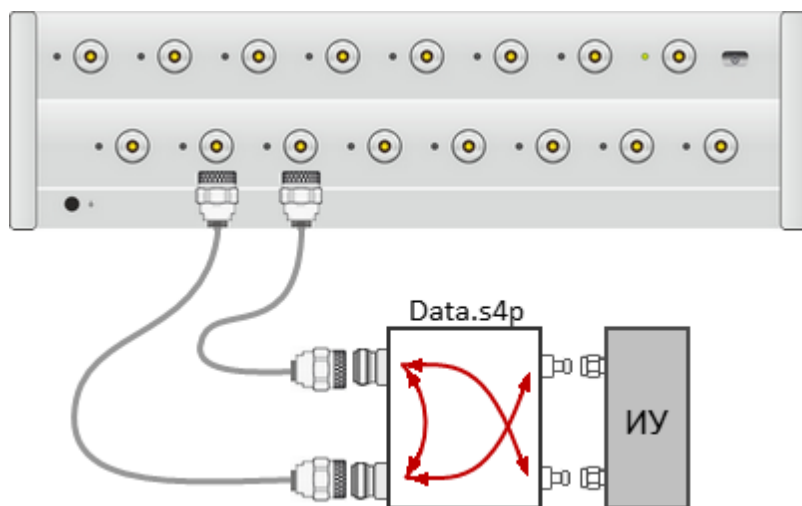
четырёхпортовое исключения/встраивания цепей
