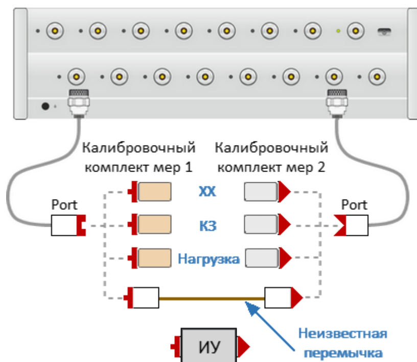
Рисунок 114 — Калибровка с неизвестной перемычкой SOLR (ИУ с разъемами различных видов)
