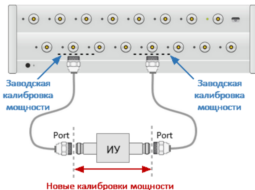
Рисунок 116 — Калибровка мощности
