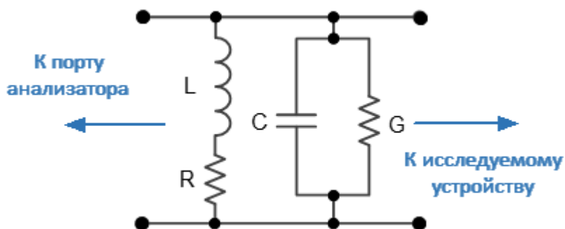
Рисунок 161 – Предустановленная согласующая цепь
