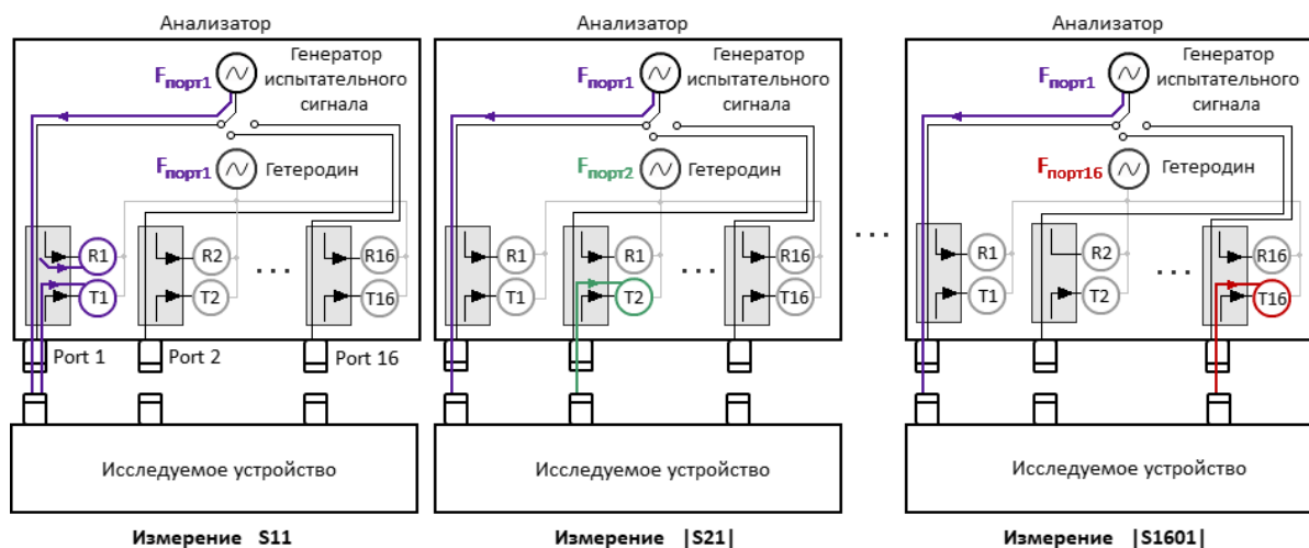
Рисунок 175 — Режим смещения частоты между портами
