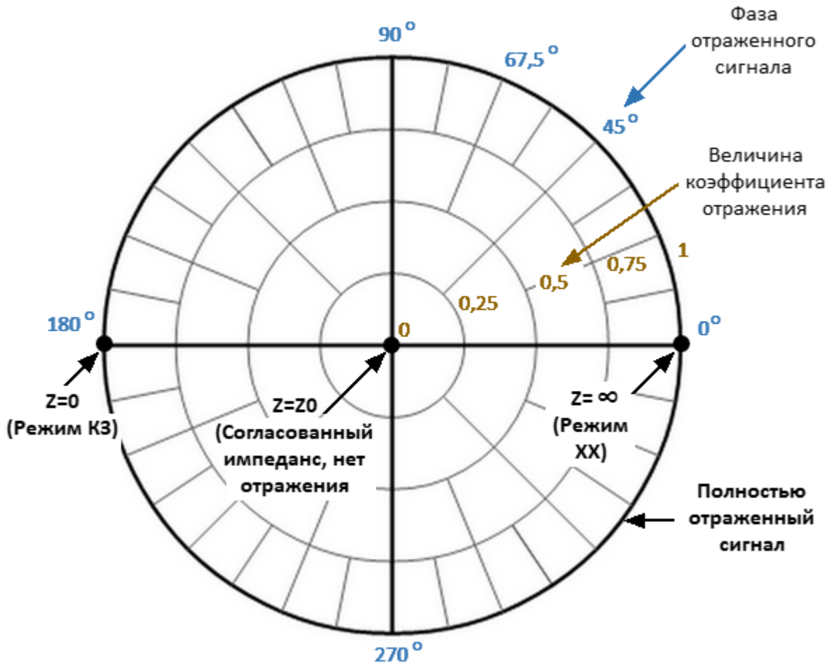
Рисунок 66 — Свойства полярной диаграммы
