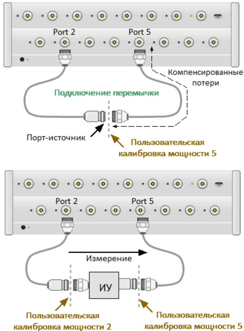
Рисунок 119 — Калибровка приёмников
