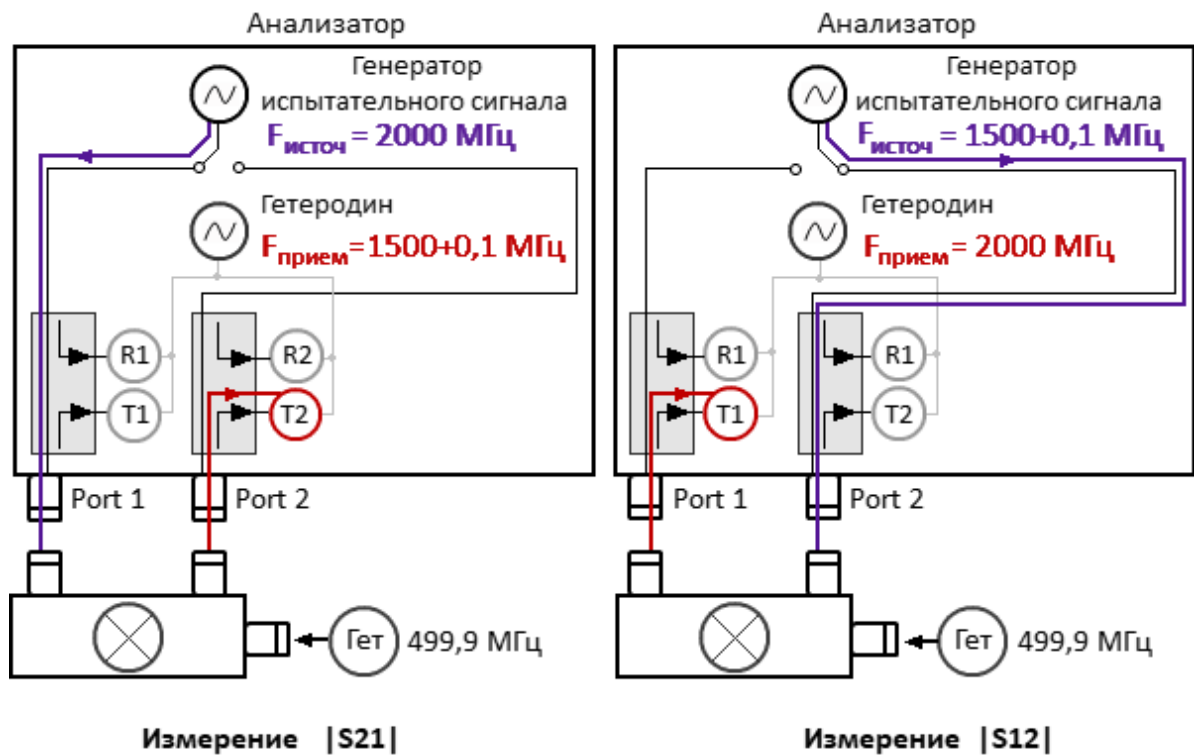
Рисунок 182 — Измерение S-параметров смесителя в режиме АПЧС с подстройкой частоты порта 2
