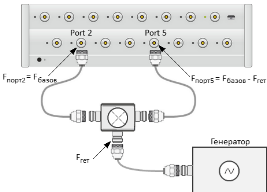
Рисунок 174 — Измерение смесителя с использованием смещения частоты
