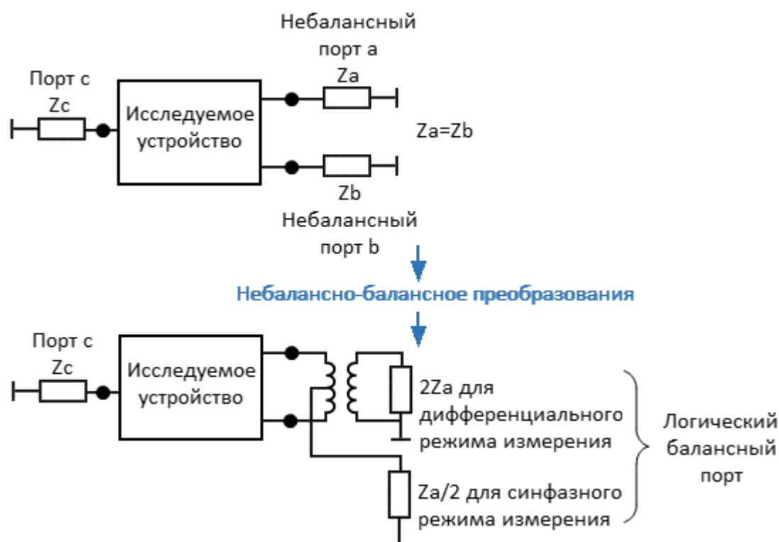
Рисунок 163 — Схема небалансно-балансного преобразования
