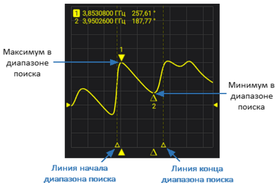
Рисунок 141 — Диапазон поиска
