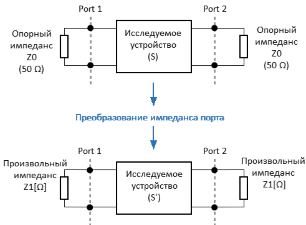
Рисунок 153 — Преобразование импеданса порта
