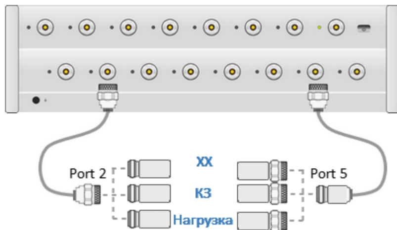
Рисунок 120 — Скалярная калибровка смесителей
