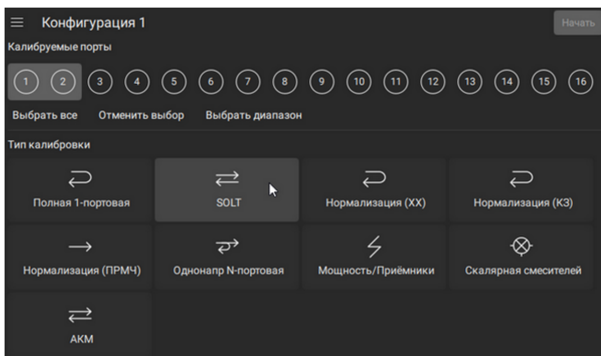
Рисунок 97 — Пример объединения портов в группу (для порта 1 и порта 2 назначается калибровка SOLT)
