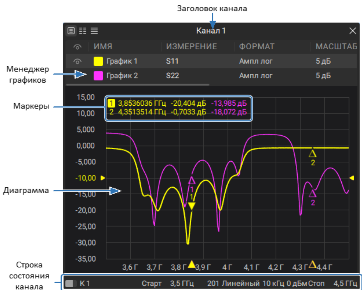
Рисунок 29 – Окно канала
