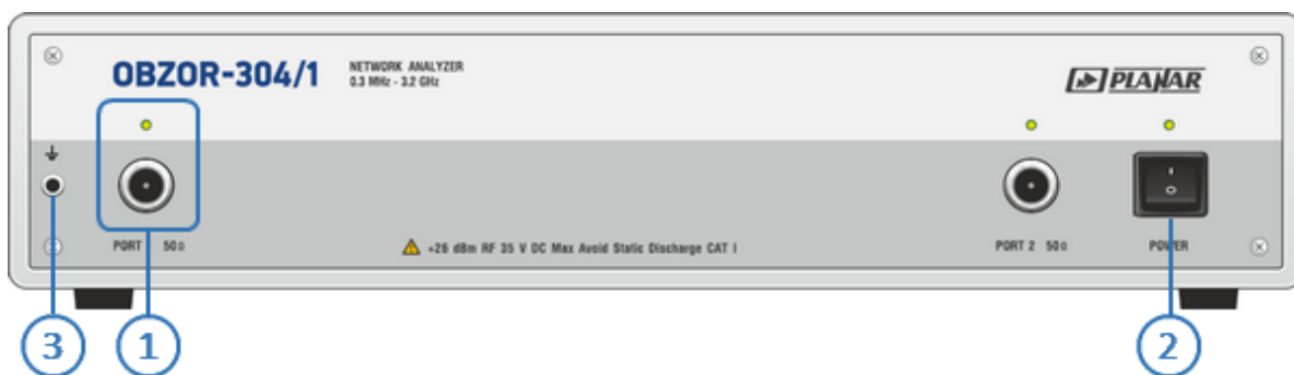
Рисунок 8 – Передняя панель
