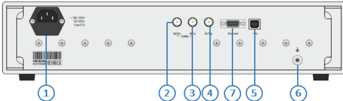
Рисунок 9 – Задняя панель
