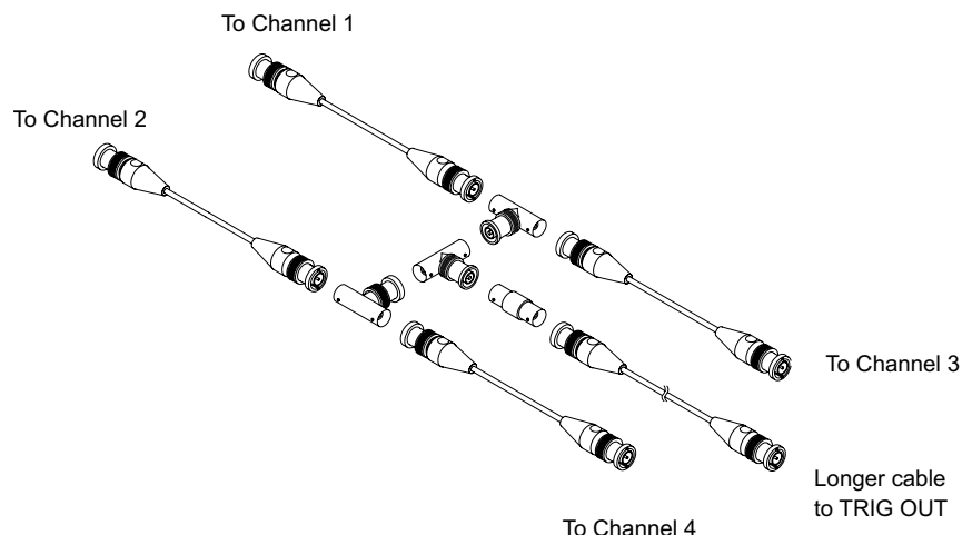
Рис. 50 Соединение кабелей для пользовательской калибровки четырехканального осциллографа
