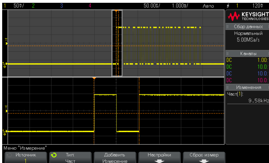
Рис. 48 Локализация события с целью измерения частоты
