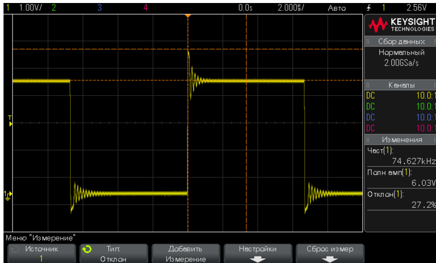
Рис. 47 Автоматическое измерение отклонения от установленного значения
