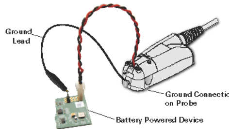
Рис. 45 Измерения на устройстве с батарейным питанием с помощью пробника N2820A
