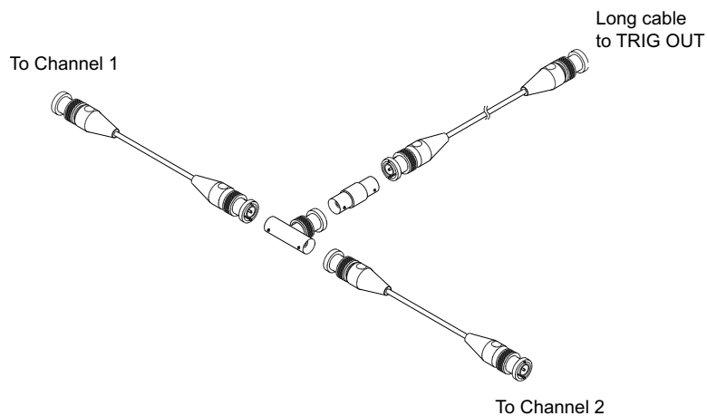
Рис. 49 Соединение кабелей для пользовательской калибровки двухканального осциллографа
