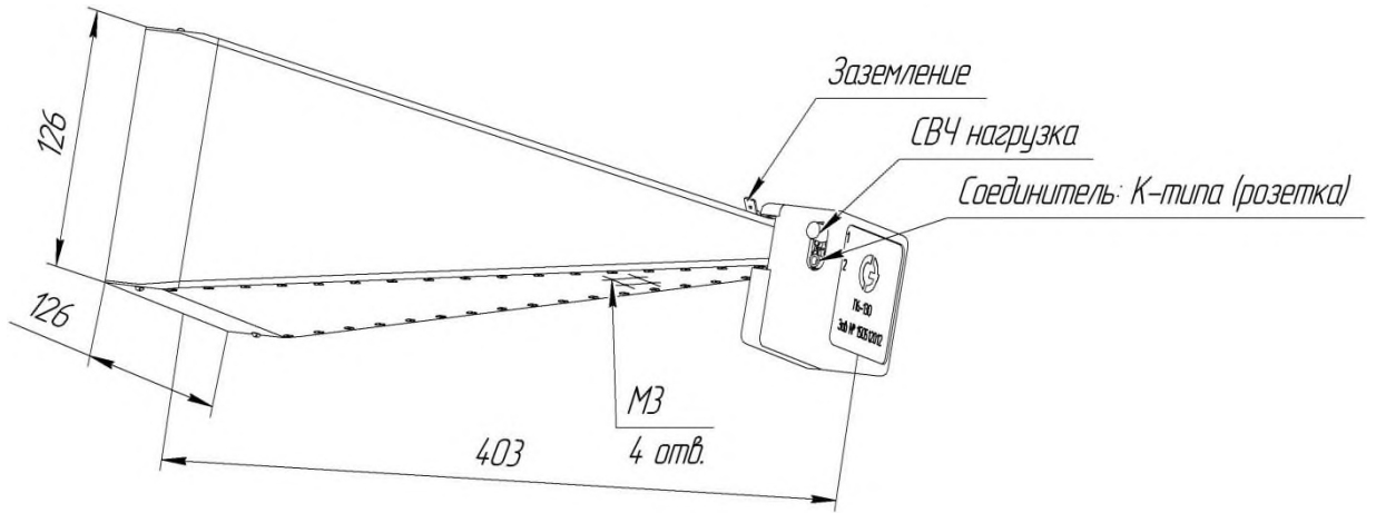
Рисунок 1 – Внешний вид рупора П6-130
