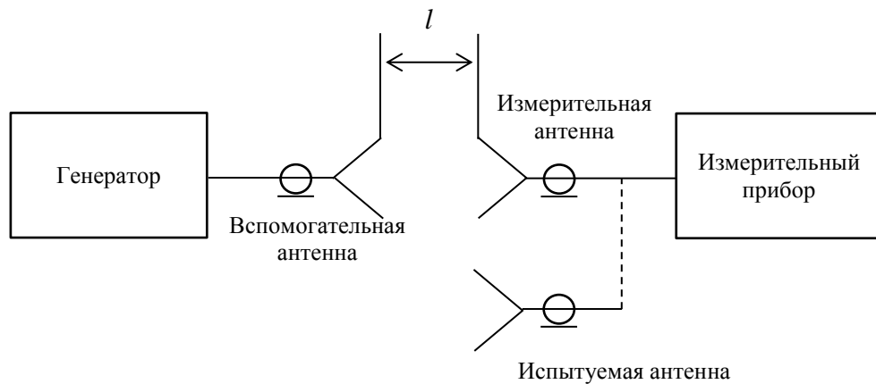
Рисунок 8 – Схема соединения приборов при измерении эффективной площади.
