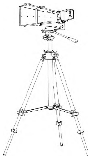
Рисунок 5 – Общий вид рупора П6-130 в развёрнутом положении
